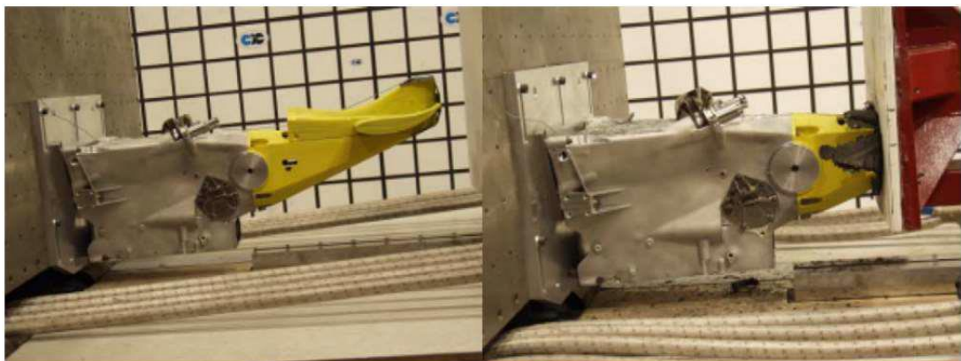
Figure 1.10. Official FIA F1 RIMP test [20].
