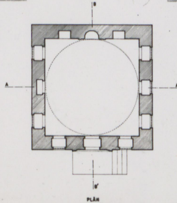
PLÂN
