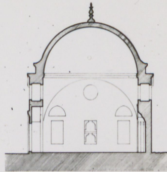
B.-B' KESİTİ
