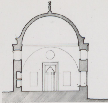
A.-A' KESİTİ
