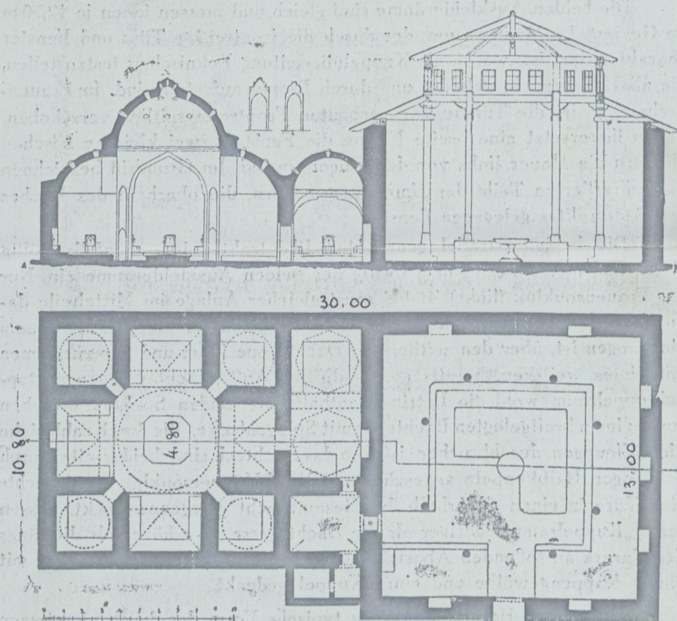
Abb. 41. Agha Hammam, Grundriß und Schnitt.
