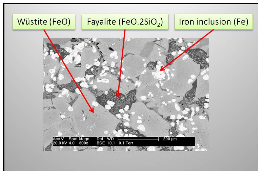
Figure 3.11. Finery slag
