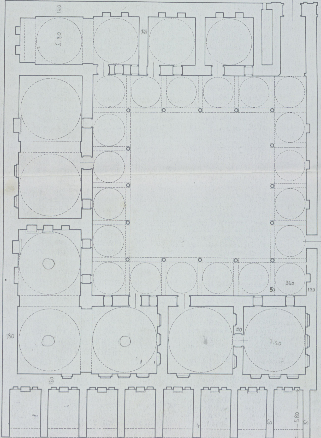
Manisa — Muradiye Külliyesi İmaretî Plân Projesi
