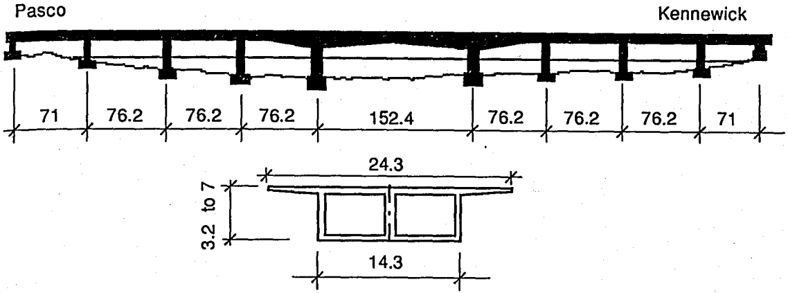
(d) CONCRETE BOX GIRDER - CANTILEVER METHOD
