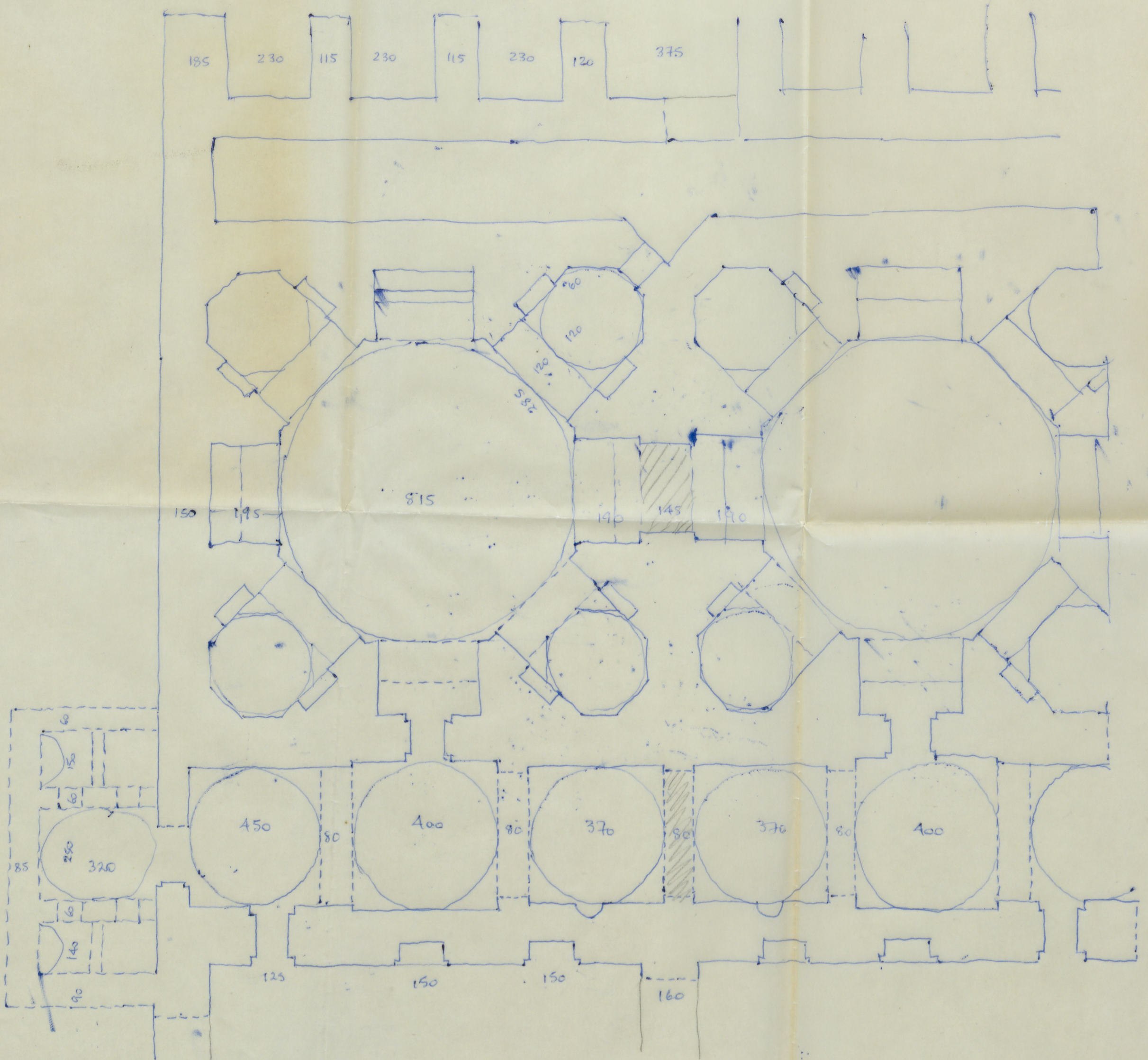
ÜSKÜDAR, VALİDE HAMAMI 1/100
