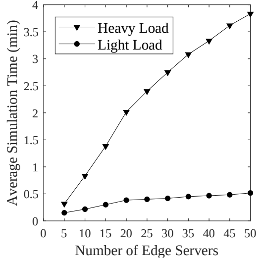
(d) Average simulation time
