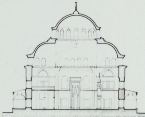
GENİSLİĞİNE KESİT
