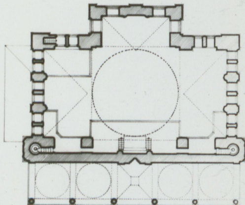
MAHFEL PLÂNI
