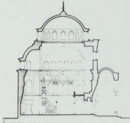
UZUNLUĞUNA KESİT
