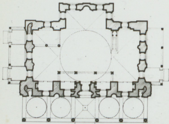
ZEMİN KAT PLÂNI
