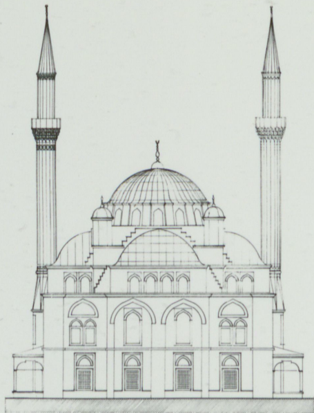
MİHRAP CEPHESİ
